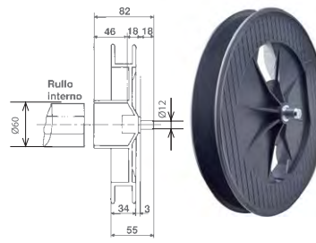
AT25001 Puleggia in PVC ø 180 mm perno sporgente € 3,15
