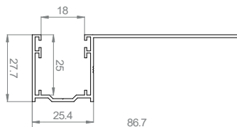
AT36017 Guida per tapparella con distanziale 65
