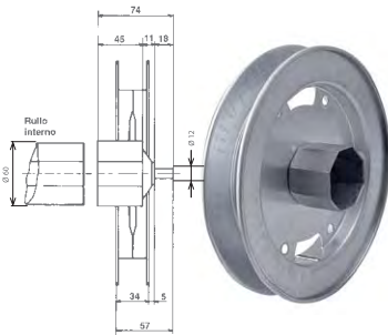
AT25004 Puleggia zincata ø 180 mm € 6,80
