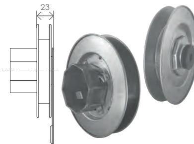
AT21008 Puleggia mini per avvolgitore per mod. "OMEGA" € 8,65
