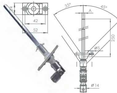
AT11007 Snodo per astina € 28,15
