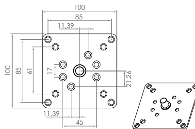
MAT014 Staffa di fissaggio per motori con manovra di soccorso € 6,00
