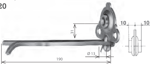
AT31002 Supporto pesante completo € 12,70
