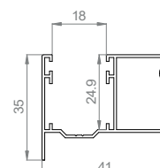
AT36015 Guida per tapparella con distanziale 20
