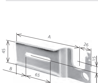
AT31014 Mensola "TORINO/PIEGA11" zincata - SX € 3,80
