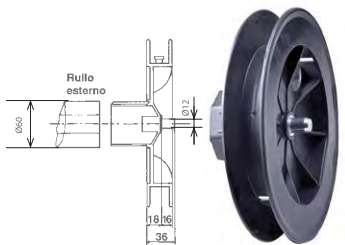
AT25013 Puleggia in PVC ø 180 mm con perno rientrato € 3,45
