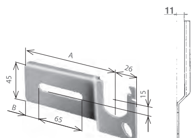
AT31013 Mensola "TORINO/PIEGA11" zincata - DX € 3,80
