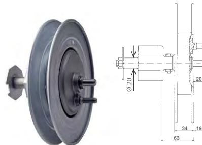
AT25007 Riduttore ZAMA "A/63-220" Kg. 40 € 57,80
