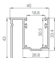
AT36001 Guida per tapparella con distanziale 17
