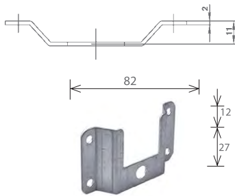
AT31008 Supporto a legno € 1,10
