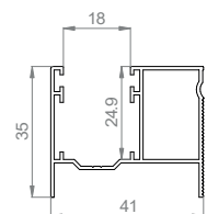
AT36015 Guida per tapparella con distanziale 20
