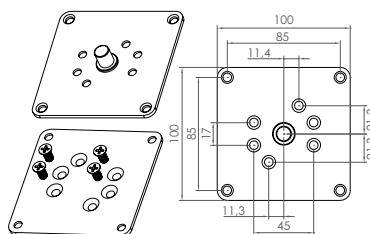
MAT012 Staffa di fissaggio per motori con manovra di soccorso, su richiesta per ridurre l'ingombro € 7,00
