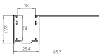
AT36017 Guida per tapparella con distanziale 65
