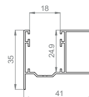
AT36015 Guida per tapparella con distanziale 20
