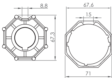
MATS06 Adattatore per rullo \varnothing 59 mm ottagonale da 70 mm € 9,00
