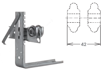
AT31005 Supporto regolabile con cuscinetto per bifora € 31,25
