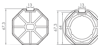
MATS04 Adattatore per rullo ottagonale da 70 mm ø45 mm € 8,00
