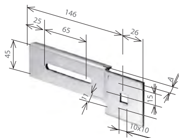
AT31022 Mensola "Torino" foro quadro € 3,75
