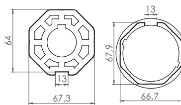
MATS07 Adattatore per rullo ottagonale \varnothing 59 mm da 70mm - di serie € 10,00
