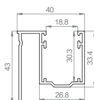
AT36001 Guida per tapparella con distanziale 17
