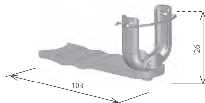
AT31003 Supporto "a murare" pesante € 9,40
